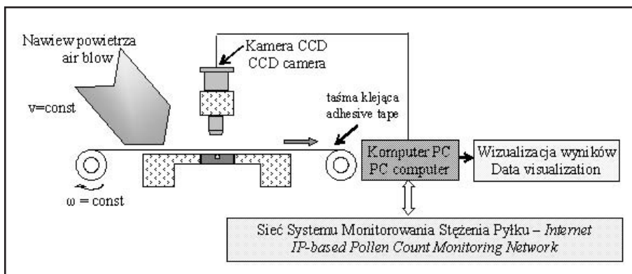
Ryc. 1. Poglądowy schemat funkcjonalny identyfikacji ziaren pyłku do monitorowania aeroalergenów. Fig. 1. Functional scheme of pollen grain identification system for aeroallergens monitoring purpose.
